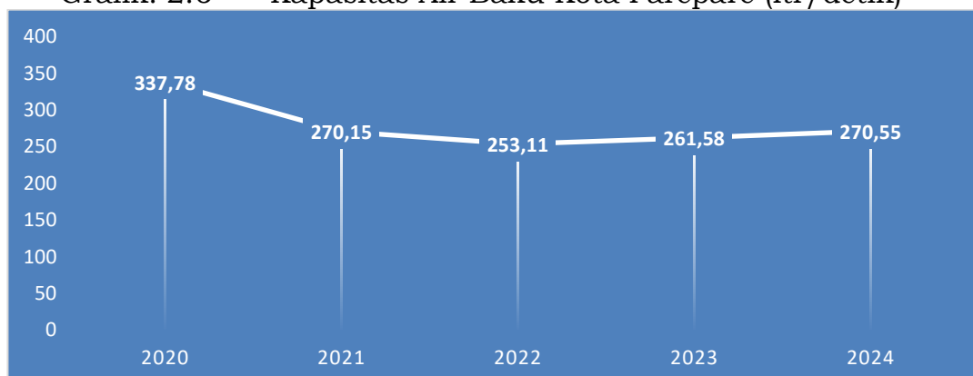
Grafik. 2.6 Kapasitas Air Baku Kota Parepare (ltr/detik)
