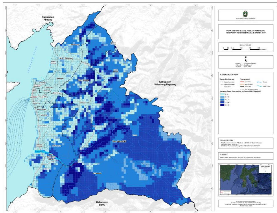
Gambar 16. Peta Ambang Ketersediaan Air Total Tahun 2030 Sumber: Hasil Analisis Tim Pokja KLHS RPJMD Kota Parepare, 2024
