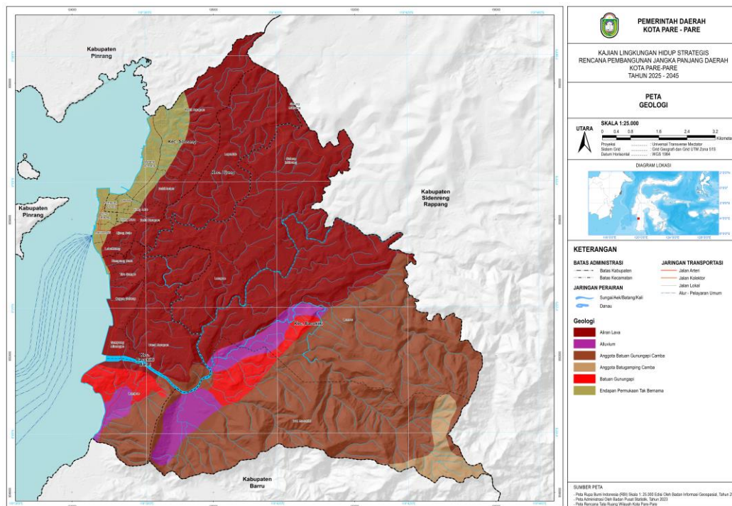
Gambar 2.5 Peta Geologi Wilayah Kota Parepare
