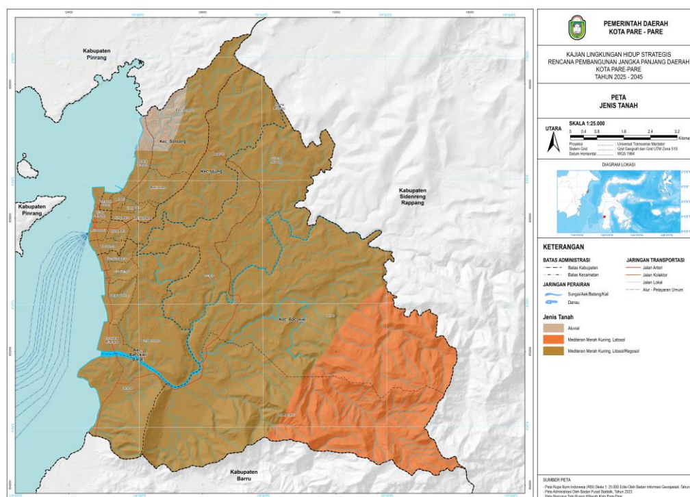
Gambar 2.4 Peta Jenis Tanah Kota Parepare
